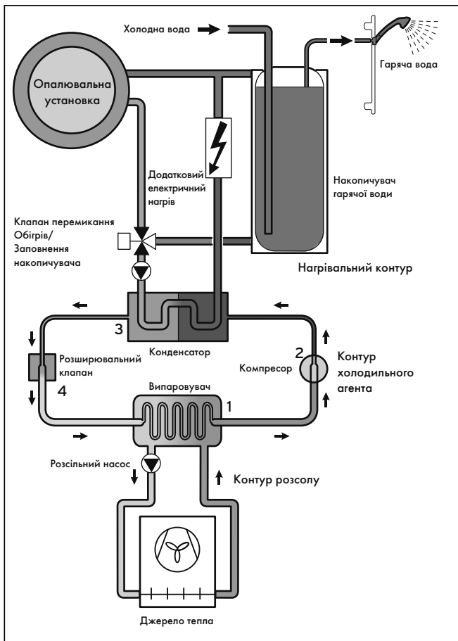
Мал. 3.4 Принцип дії теплового насоса
