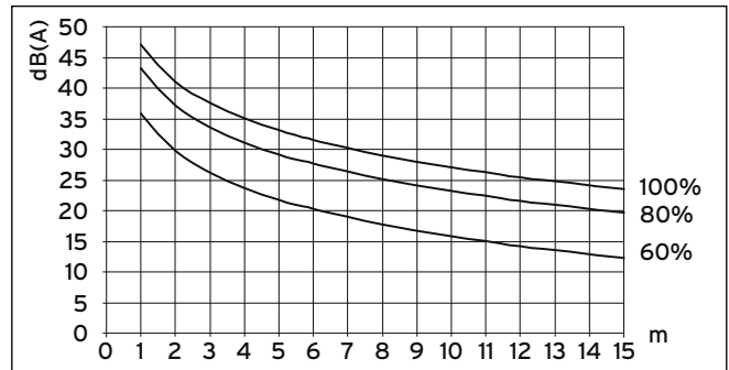
Мал. 6.1 Рівень звукового тиску зовнішнього модуля в дБ(A) залежно від віддаленості й числа оборотів вентилятора для VWL 62/3 S при установці у вільному звуковому полі
