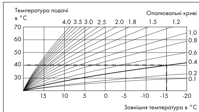
Мал. 1 Діаграма опалювальних кривих
