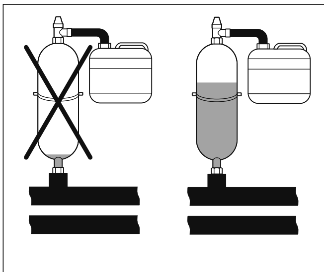
Мал. 6.4 Рівень наповнення компенсаційного резервуару для розсолу
