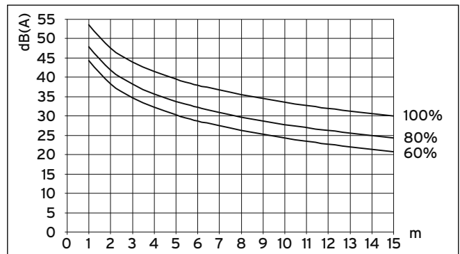
Мал. 6.2 Рівень звукового тиску зовнішнього модуля в дБ(A) залежно від віддаленості й числа оборотів вентилятора для VWL 82/3 S при установці у вільному звуковому полі
