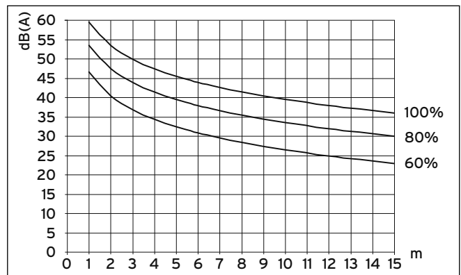
Мал. 6.3 Рівень звукового тиску зовнішнього модуля в дБ(A) залежно від віддаленості й числа оборотів вентилятора для VWL 102/3 S при установці у вільному звуковому полі
